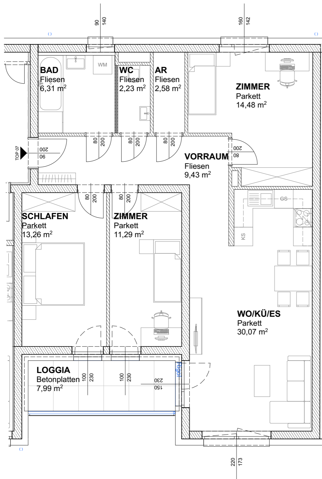
GRUNDRISS | M 1:75
